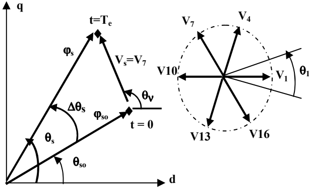
Fig. 3 : Flux deviation
