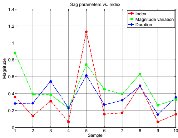
Fig. 19: Parameters Sag vs.. Indicator
