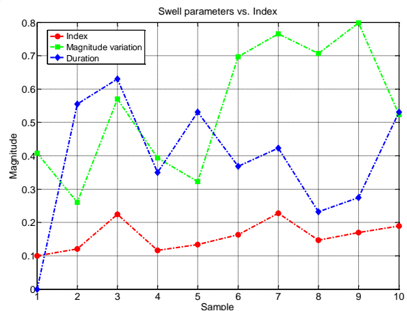
Fig. 17: Parameters vs Swell . Indicator
