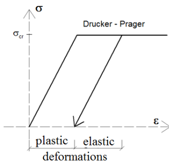
Fig. 2 Drucker-Prager model, elastic-plastic material
